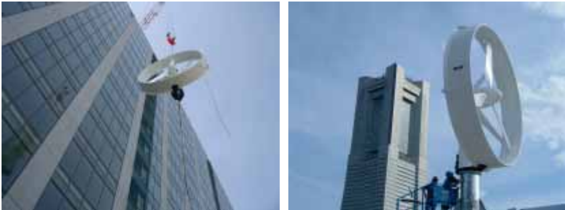
横浜市みなとみらい MM33 プロジェクトビル屋上に設置された GHDWT-10kW
